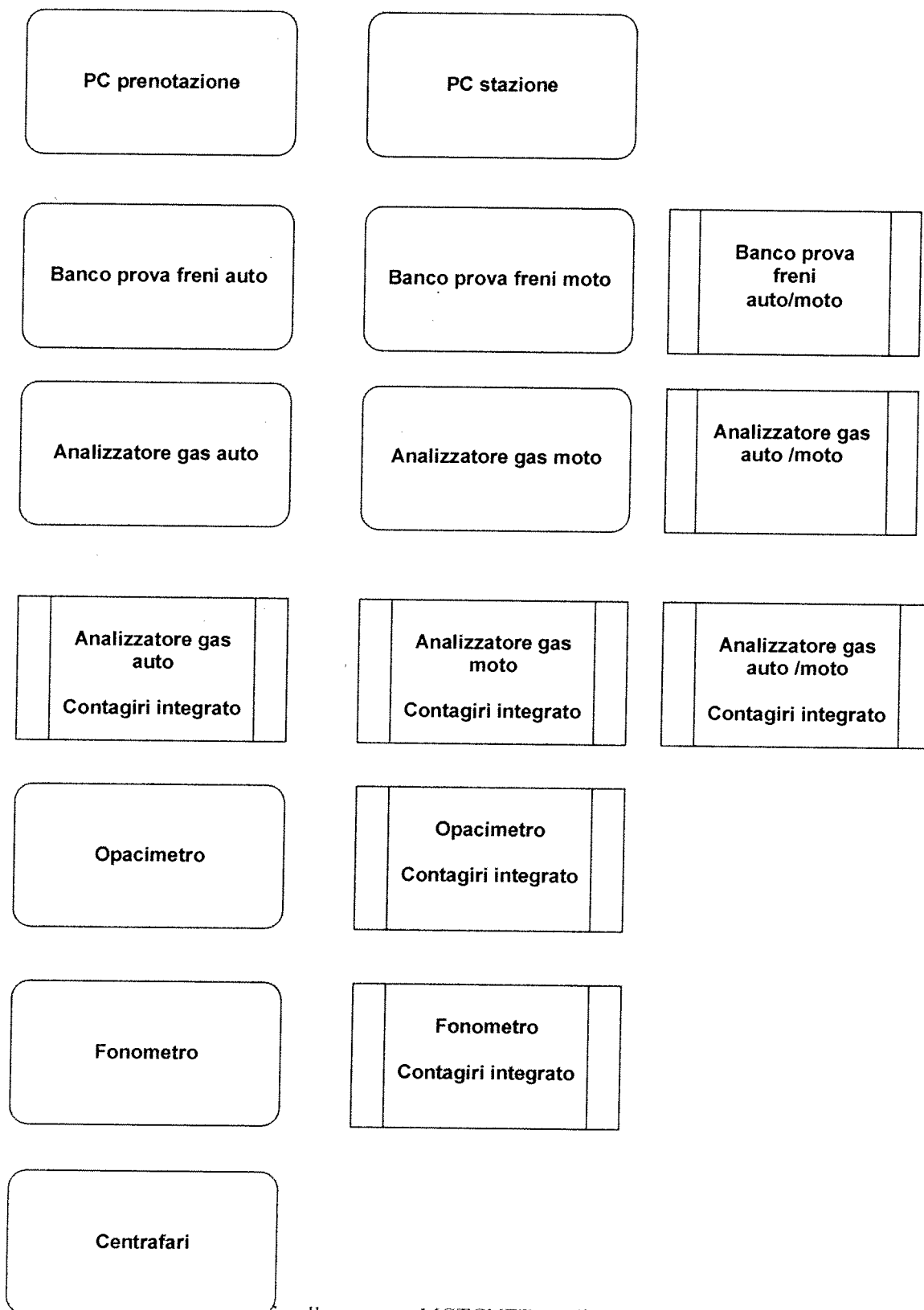
Fig. 10 - Schema di collegamento MCTCNET per linea di revisione"
